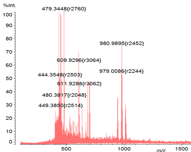
Рисунок 5S. Масс-спектр смеси \beta -октаалкорзамещенных порфиринатов Co(II) и Co(III).
