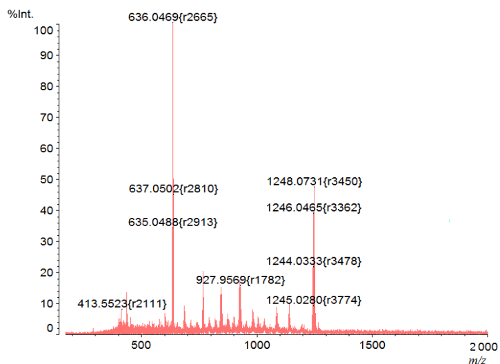
Рисунок 6S. Масс-спектр 2,3,7,8,12,13,17,18-октабром-5,10,15,20-тетрафенилпорфирина.
